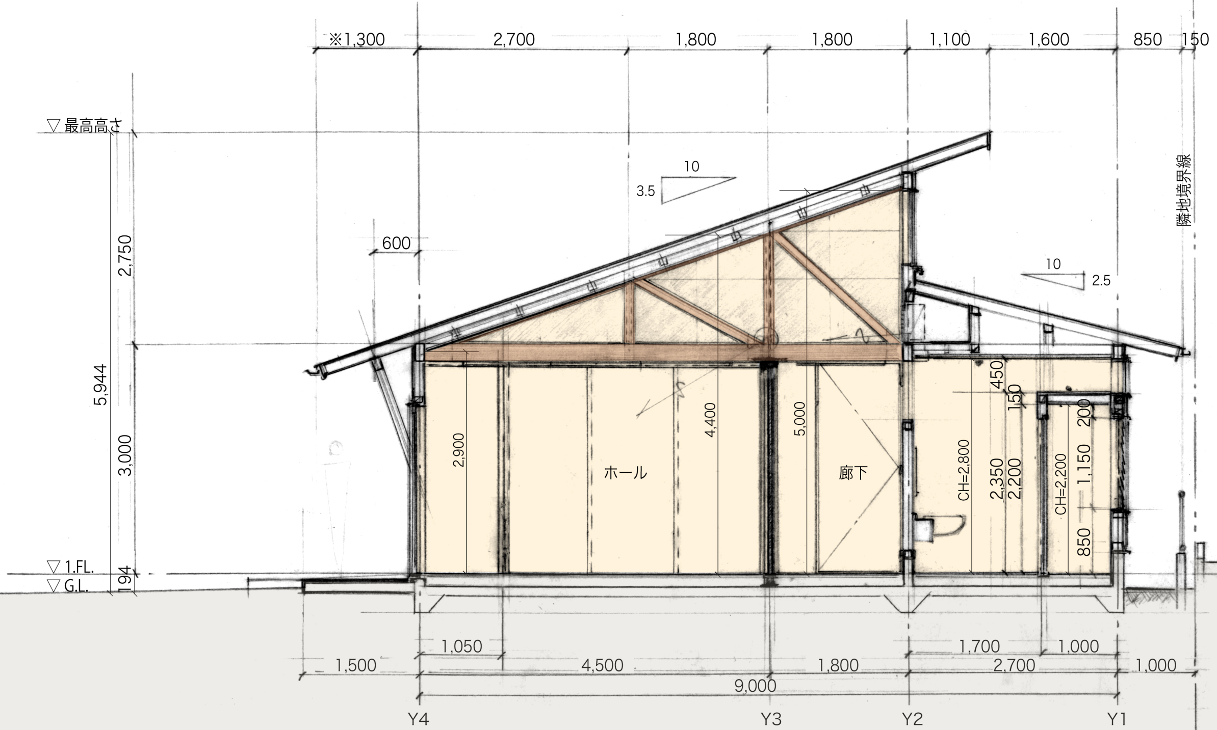
矩計図
